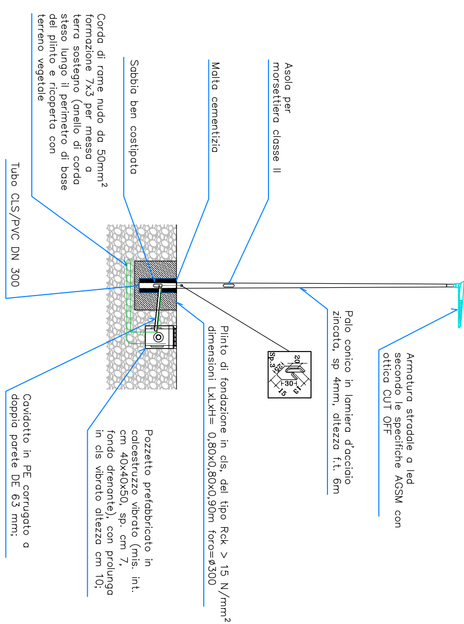
Particolare installativo – scala 1:20
